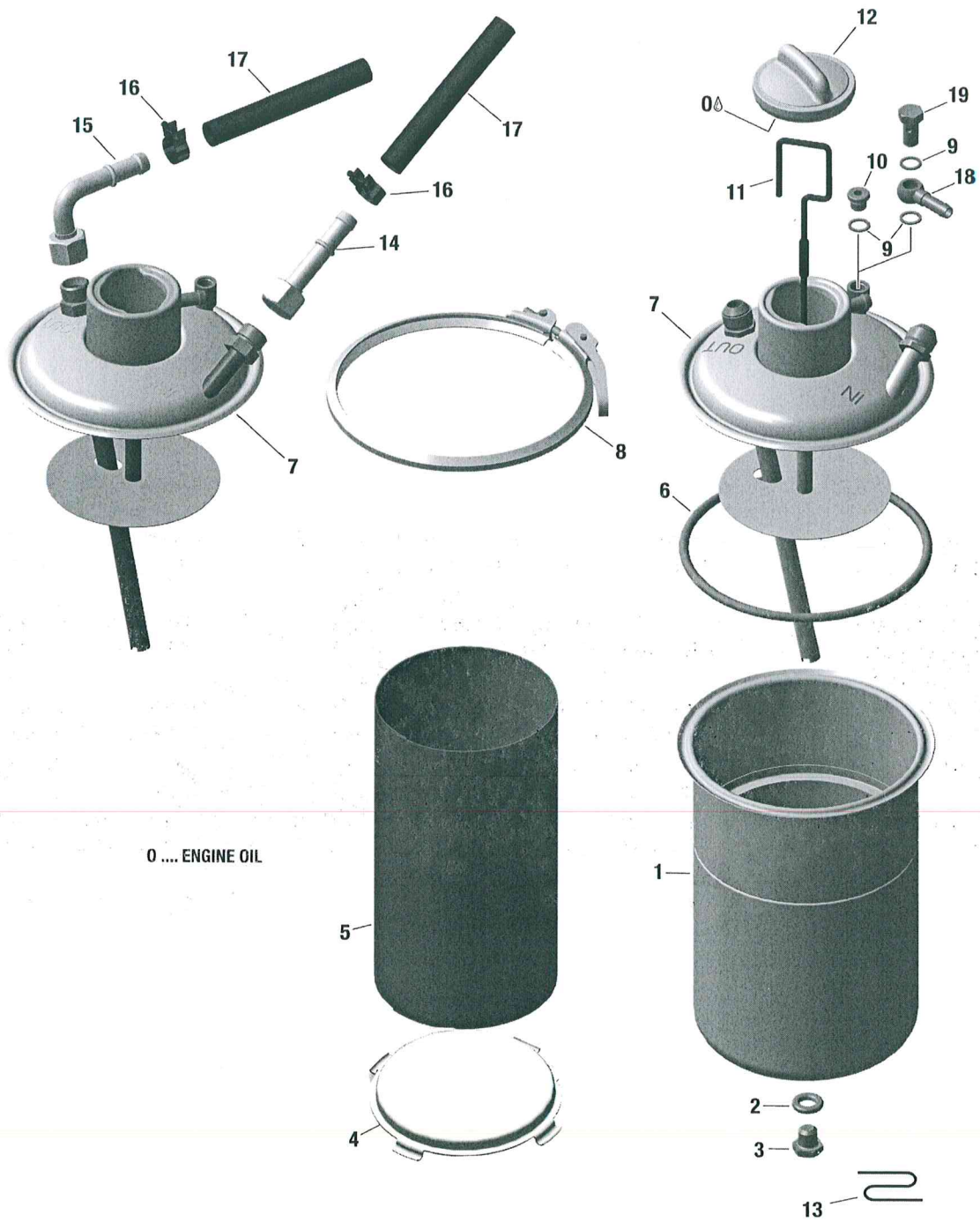
Bild/fig. 79-20-00-1
