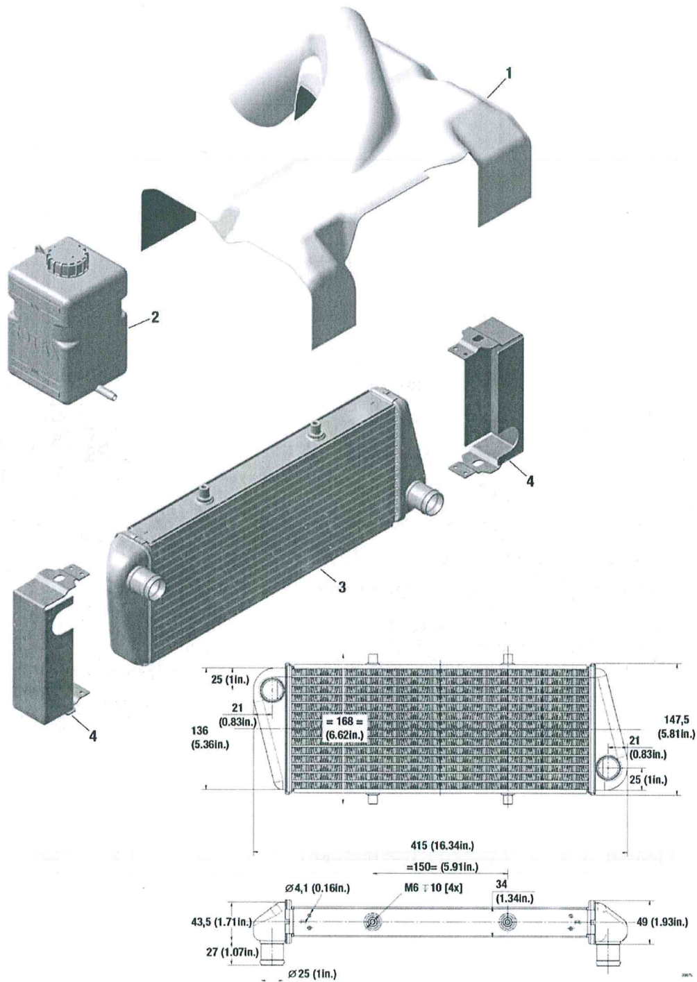
Fig. 75-20-00-3
