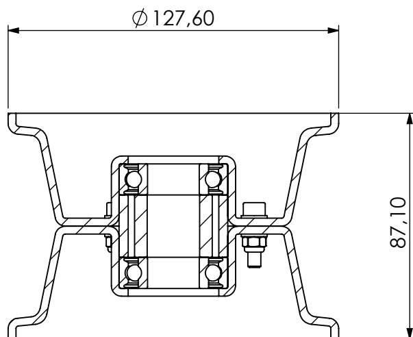
SEZIONE A-A SCALA 1 : 2
