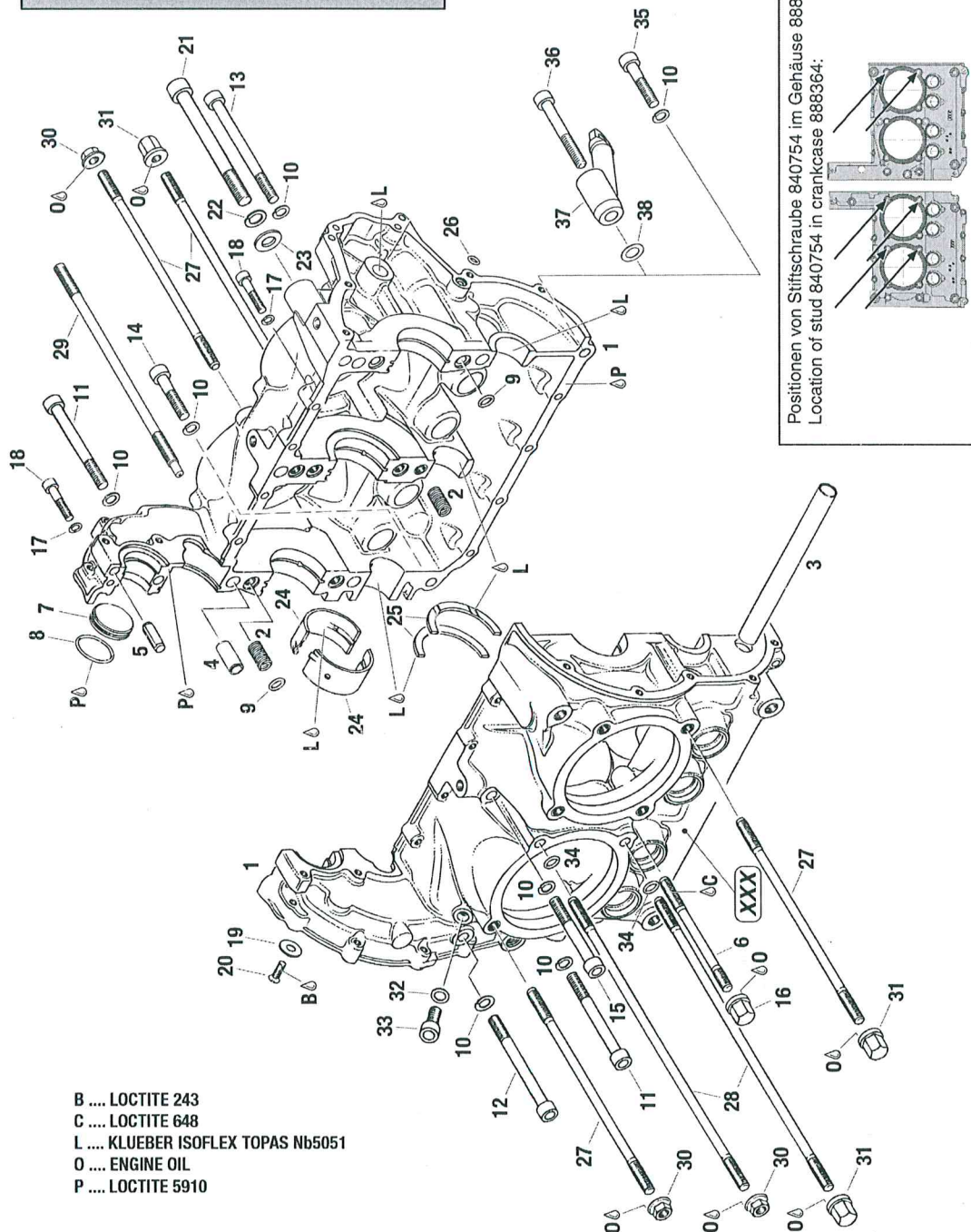
Bild/fig. 72-20-00-1
