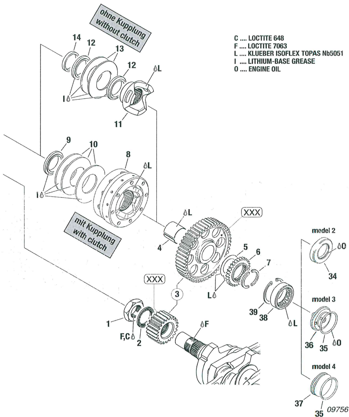
Bild/fig. 72-10-00-1
