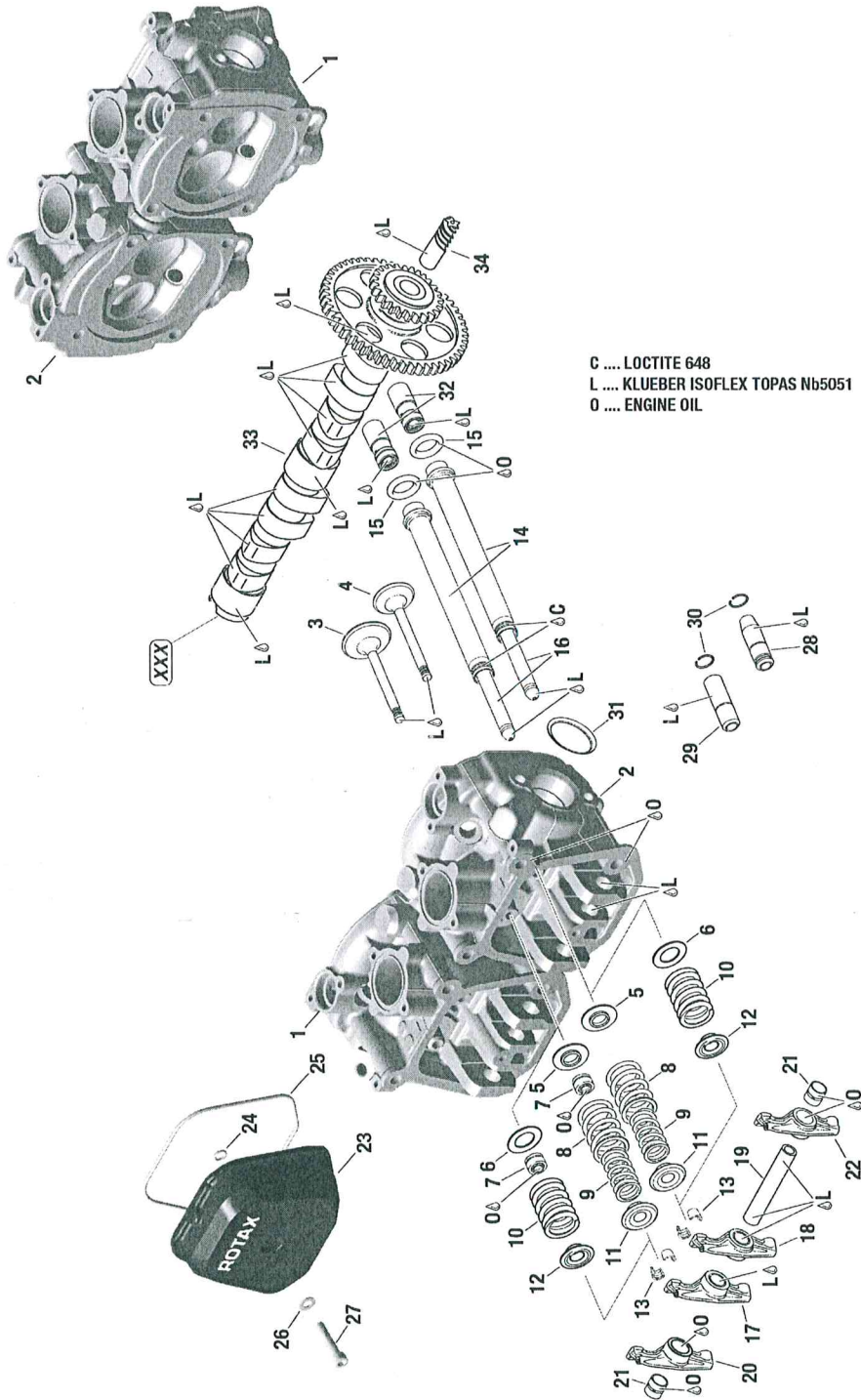
Bild/fig. 72-20-00-5
