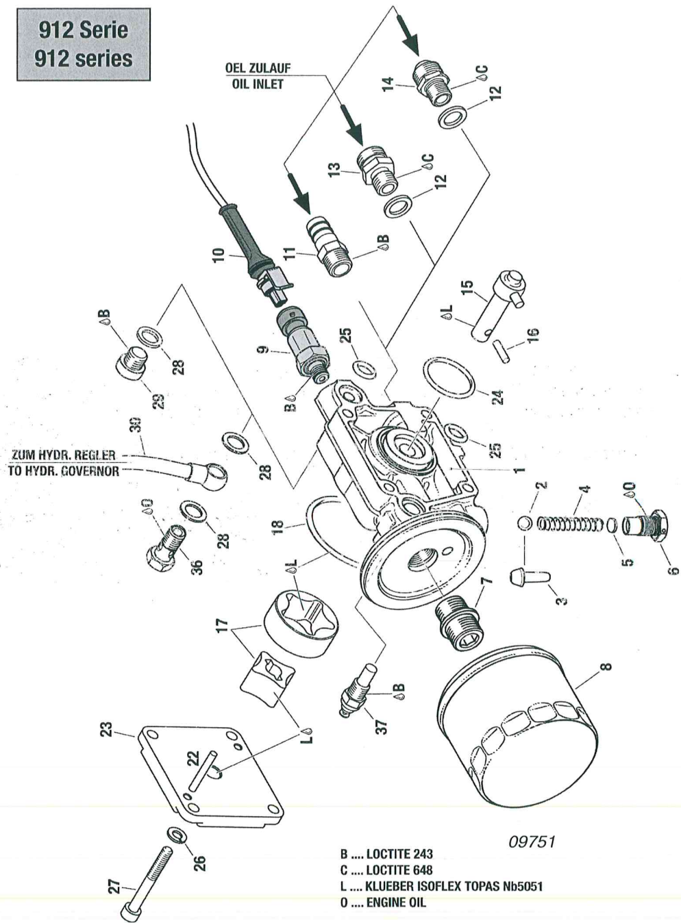
Bild/fig. 79-20-00-2
