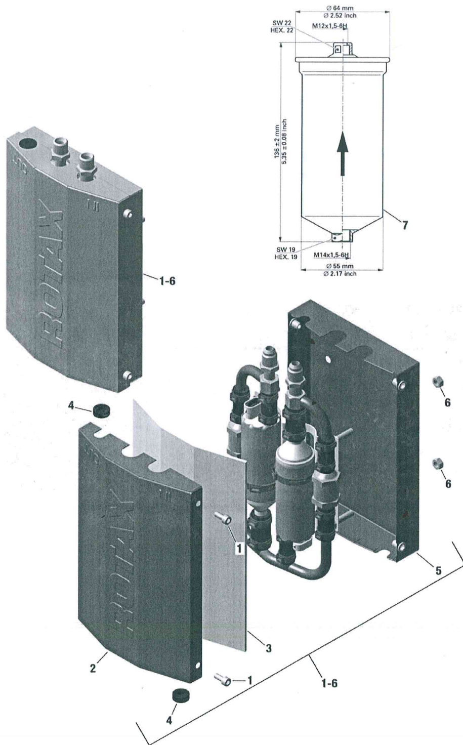
Fig. 73-10-00-4
