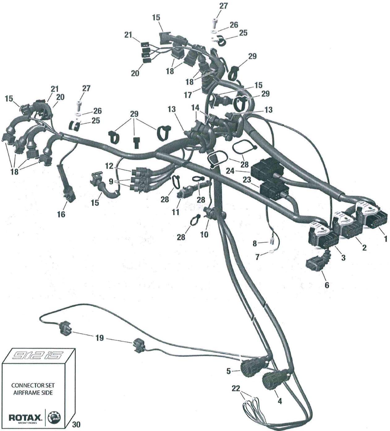
Fig. 76-50-00-1
